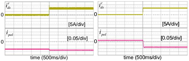
그림 3. 신호를 주입하면서 D 축 전류를 변화시켰을 때의 파형
