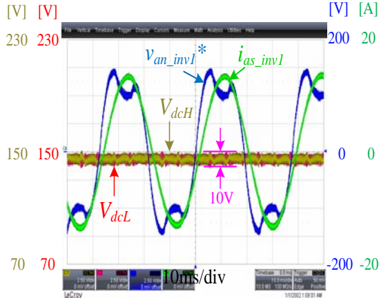
그림 2 2500W 중성점 전위 균형 제어 실험 결과 Fig. 2 Experiment Result of 2500W Neutral Point Voltage Balance Control
