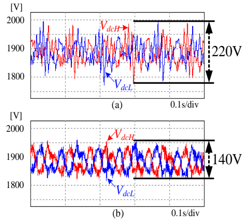
그림 3 모의 실험시 직류단 캐패시터 전압 변동 : (a) 1 개 모듈 운전시 (b) 3 병렬 운전시 Fig. 3 Simulation result of Fluctuations of DC-link capacitors : (a) 1 module operation (b) 3 parallel operation
