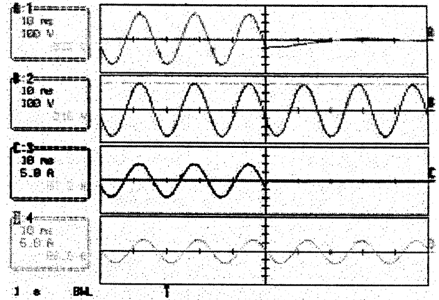
그림 13 R-L 선형부하시 응답(3KW) 확대 Fig. 13 Enlarged Response of R-L linear load(3KW)
