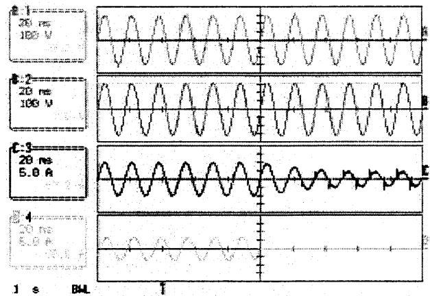
그림 9 R-L 선형부하시 응답(3KW→무부하) Fig. 9 Response of R-L linear load(3KW→No-load)
