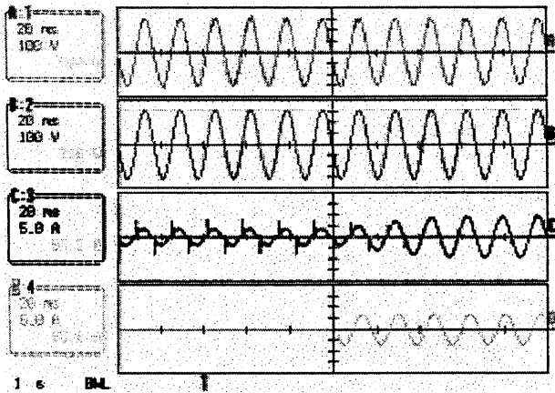
그림 10 R-L 선형부하시 응답(무부하→3KW) Fig. 10 Response of R-L linear load(No-load→3KW)
