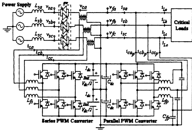
그림 5 델타 변환 UPS 시스템 구성도 Fig. 5 Delta conversion UPS system diagram
