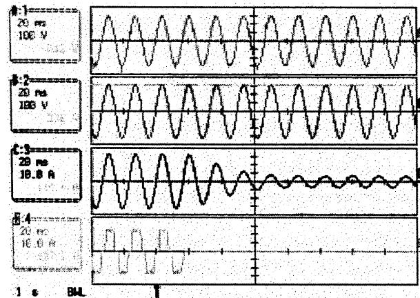
그림 11 비선형부하시 응답(63%→무부하) Fig. 11 Response of nonlinear load(63%→No-load)
