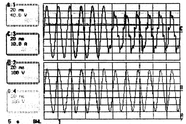
그림 15 비선형부하시 응답(63%부하) 확대 Fig. 15 Enlarged Response of nonlinear load(63% load)
