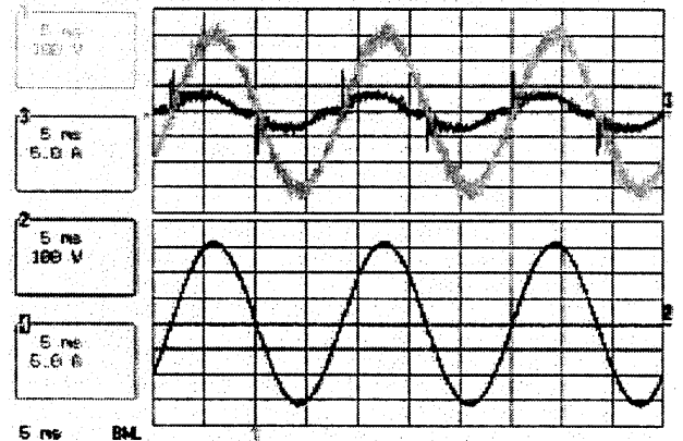
그림 8 무부하시 응답 Fig. 8 Response of No-load
