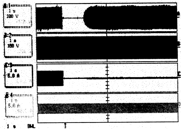
그림 12 R-L 선형부하시 응답(3KW) Fig. 12 Response of R-L linear load(3KW)
