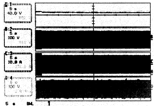
그림 14 비선형부하시 응답(63%부하) Fig. 14 Response of nonlinear load(63% load)
