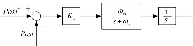
그림.4 제어기와 시스템의 모델링
