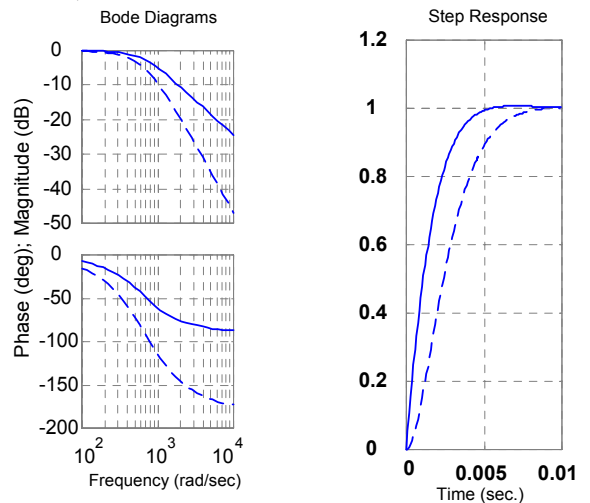
그림.7 전향보상이 없는 경우(점선) 속도 전향보상의 경우(실선)
