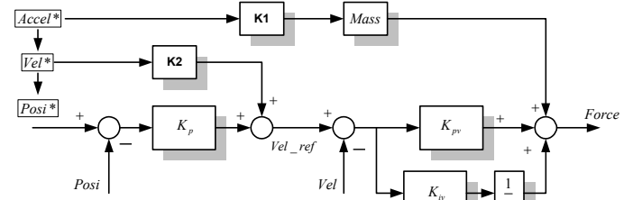
그림.5 전향보상을 통해 구성된 P-PI 제어기
