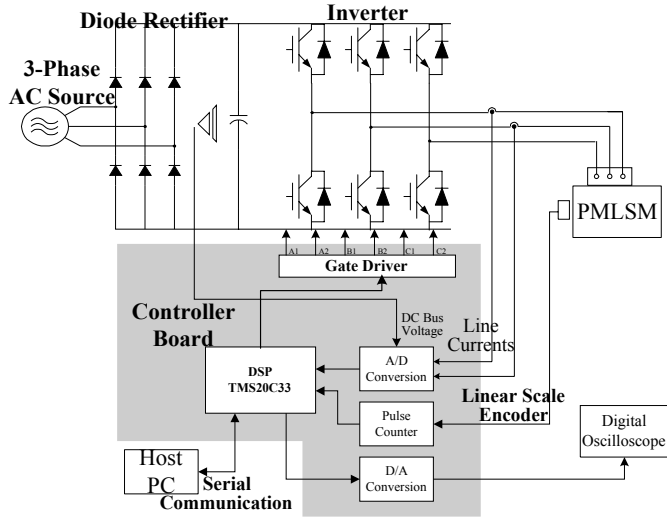
그림.8 실험장치
