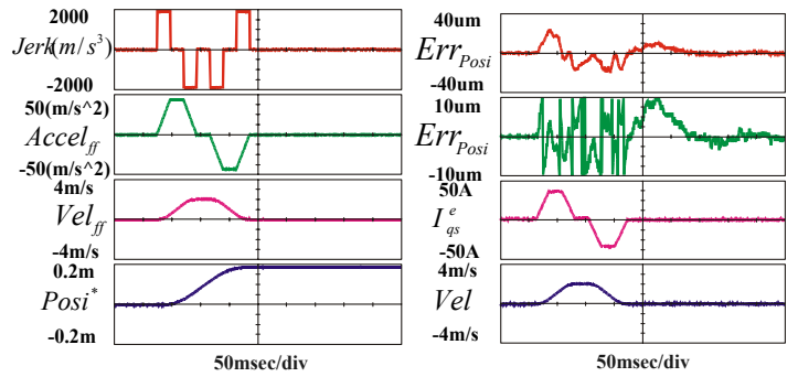
그림.10 S-Curve에 따른 위치오차와 속도 및 전류
