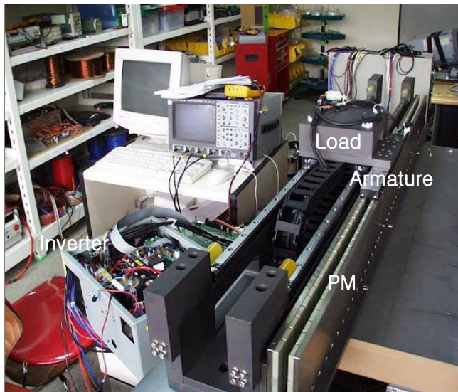
그림.9 PMLSM과 실험장비
