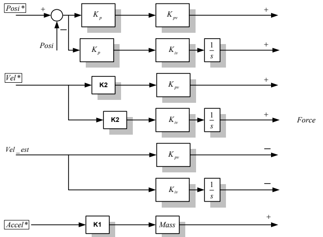
그림.6 전향보상을 통해 구성된 PID 제어기
