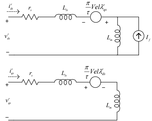
그림.1 영구자석 동기기의 동기좌표계상에서의 등가회로
