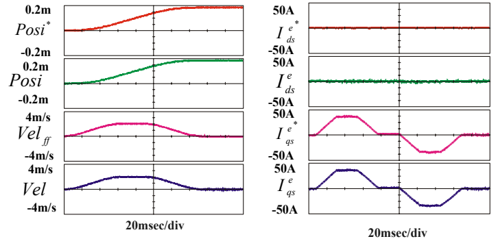
그림.11 지령값과 실제값
